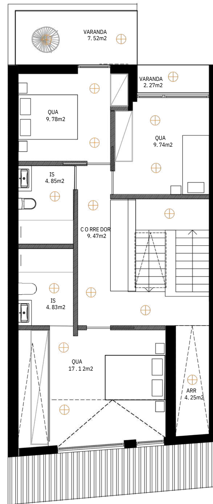
SOTÃO
